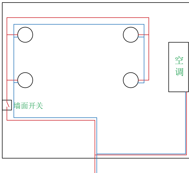
原电路
